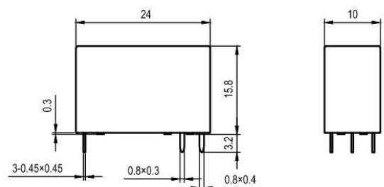
外形尺寸图
