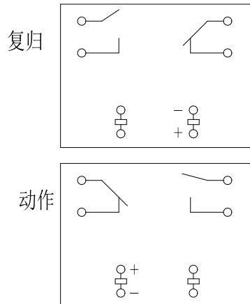
接线图
