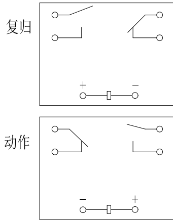
接线图
